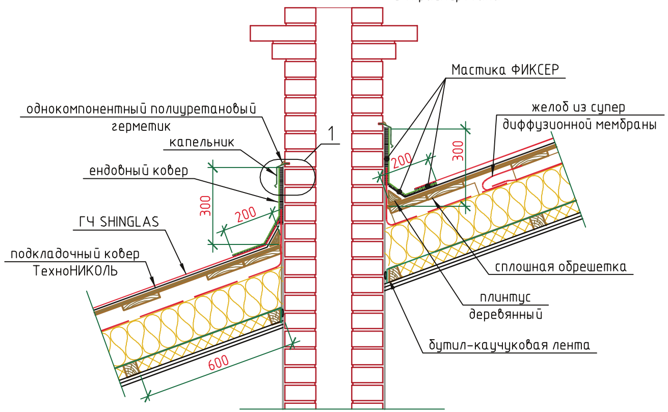
Сечение 1-1
