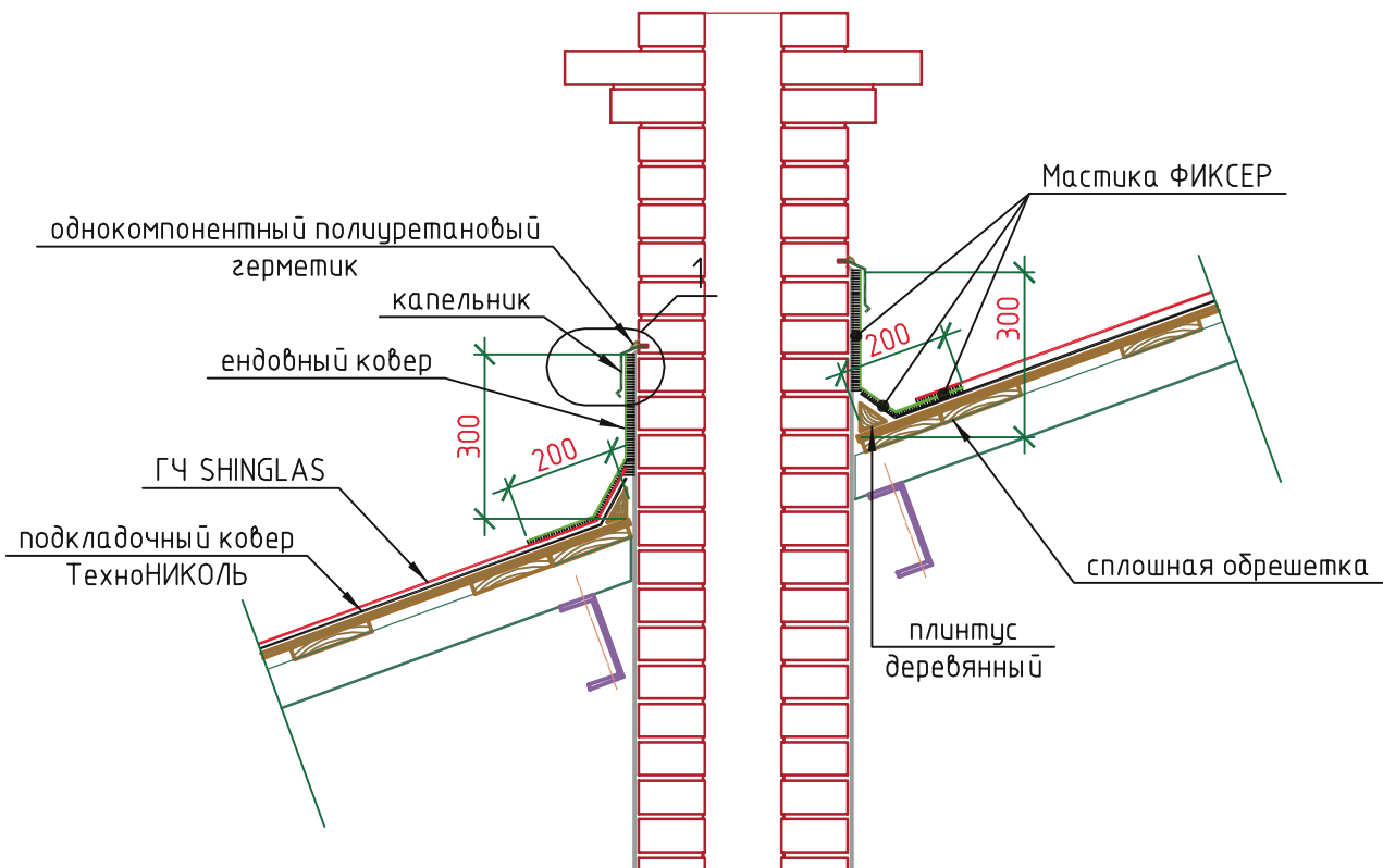
Сечение 1-1
