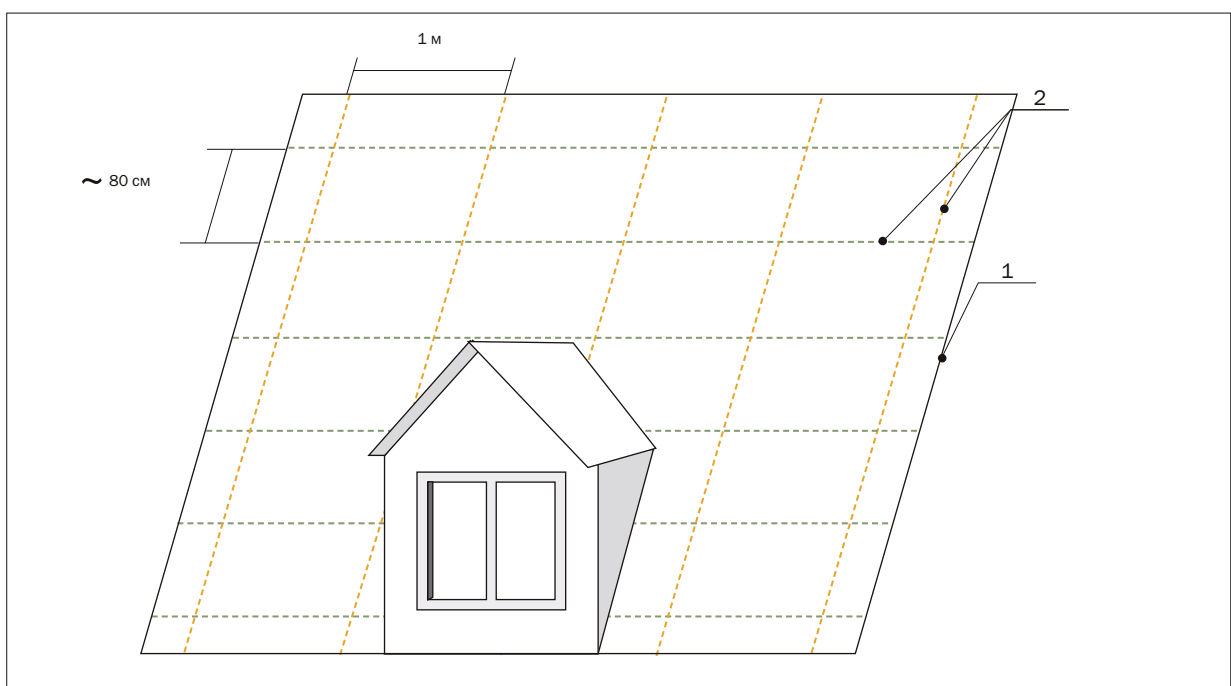
Рис. 27. Скат кровли
