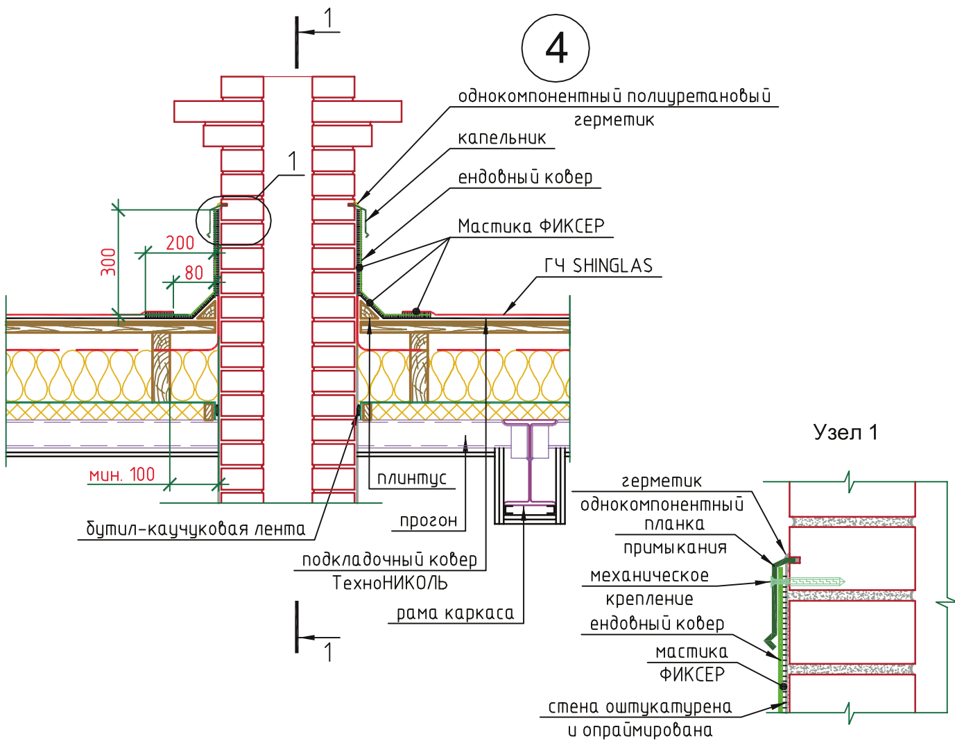
Сечение 1-1
