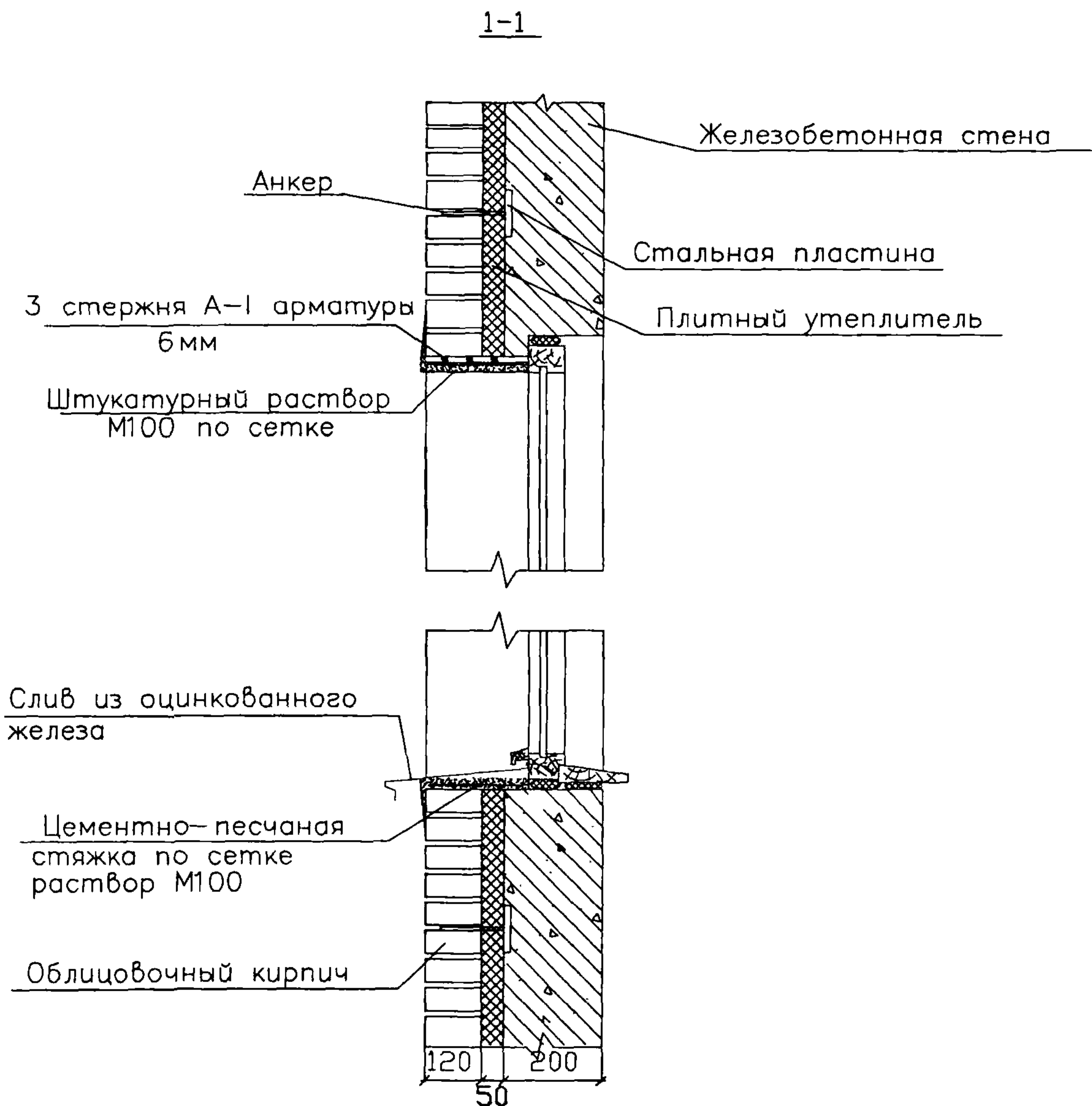
Рисунок 5 – Конструктивное решение облицовки оконных проемов
