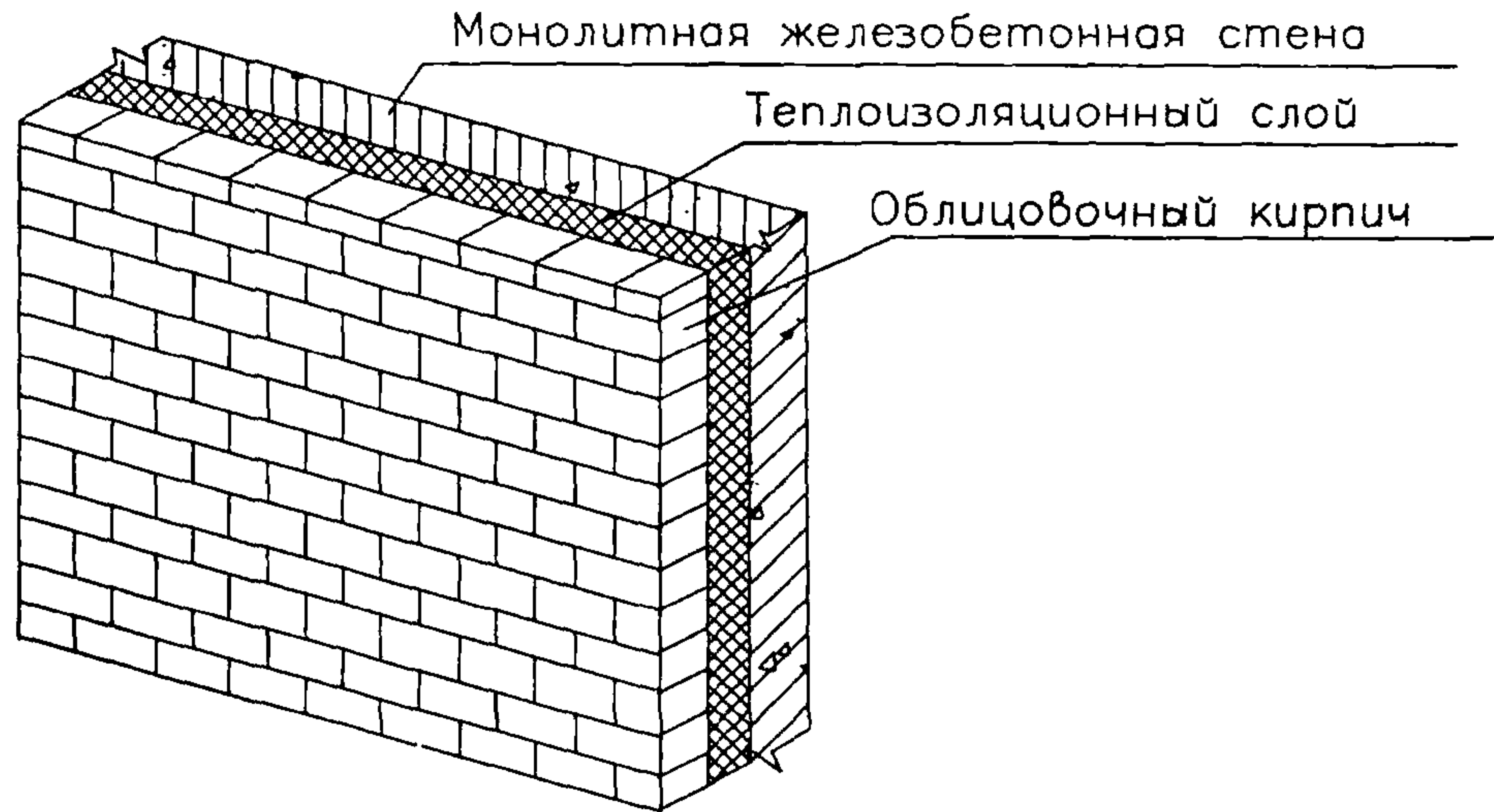
Рисунок 1 – Общий вид стены
