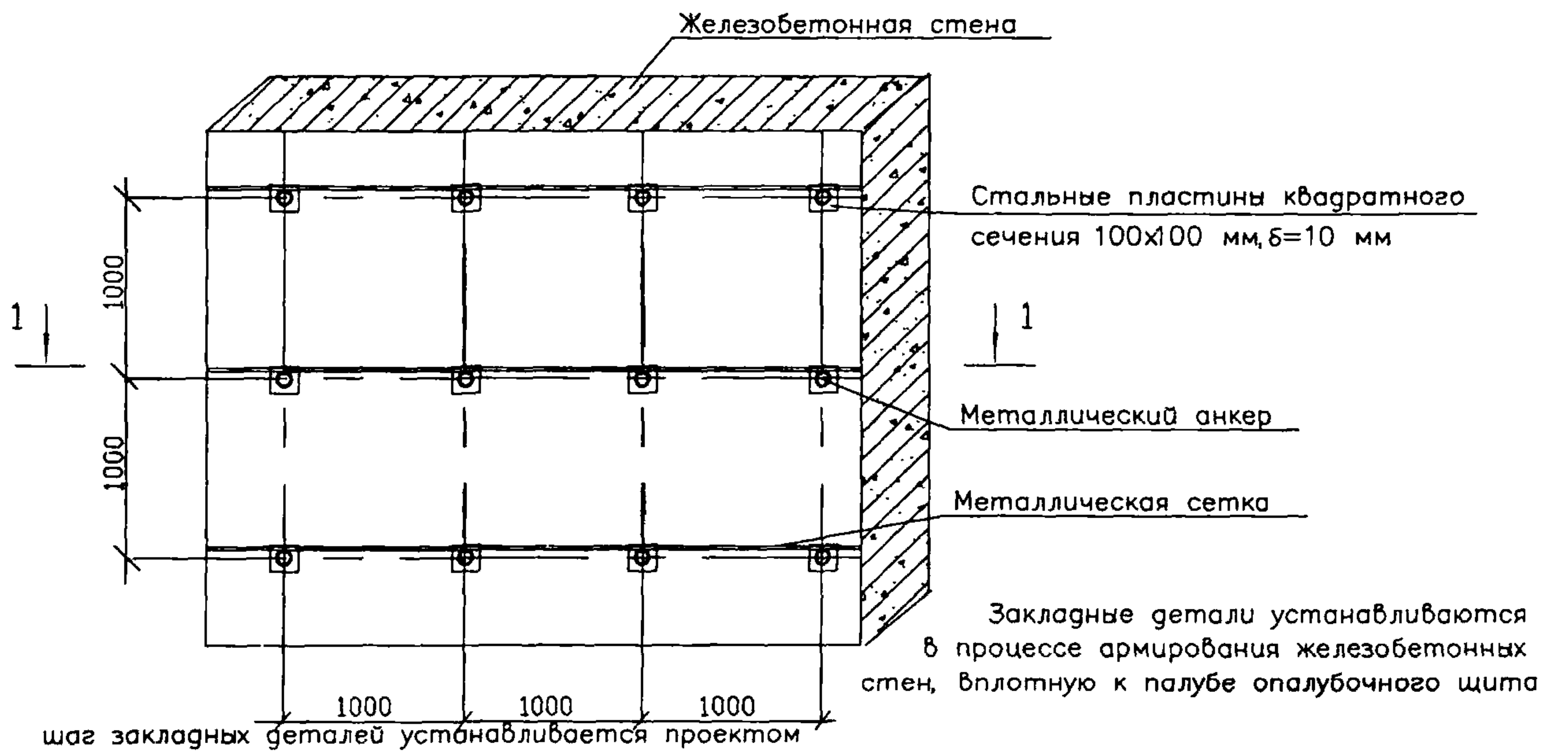
Рисунок 1 – Общий вид стены
