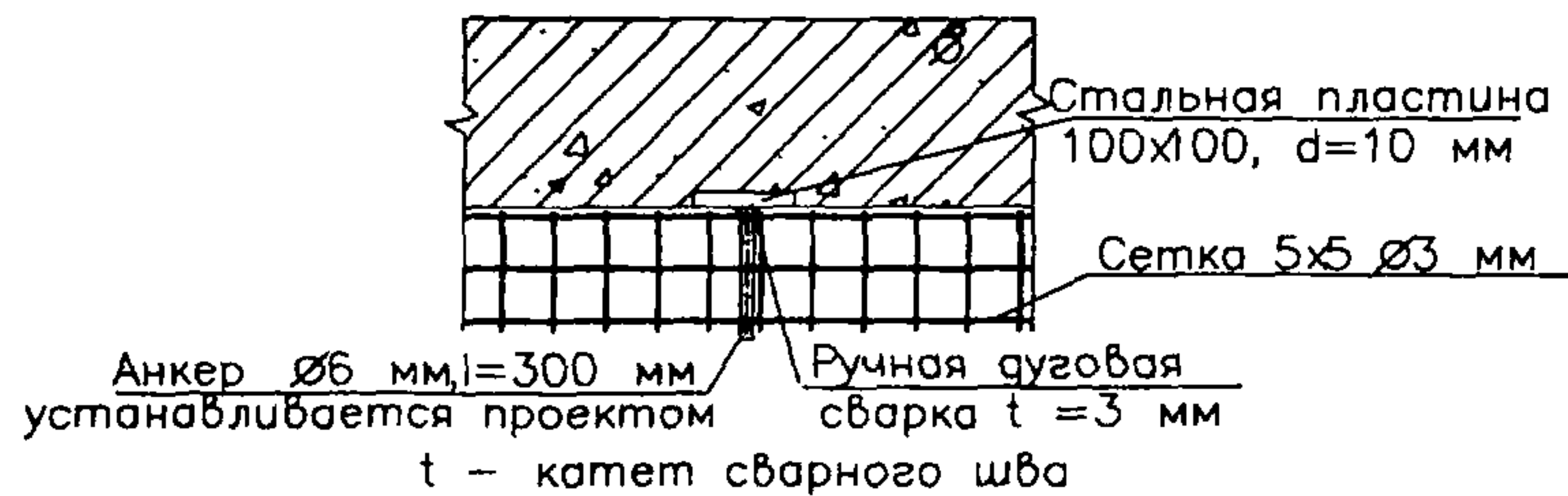
Рисунок 2 – Схема расстановки закладных деталей, устройства металлических анкеров
